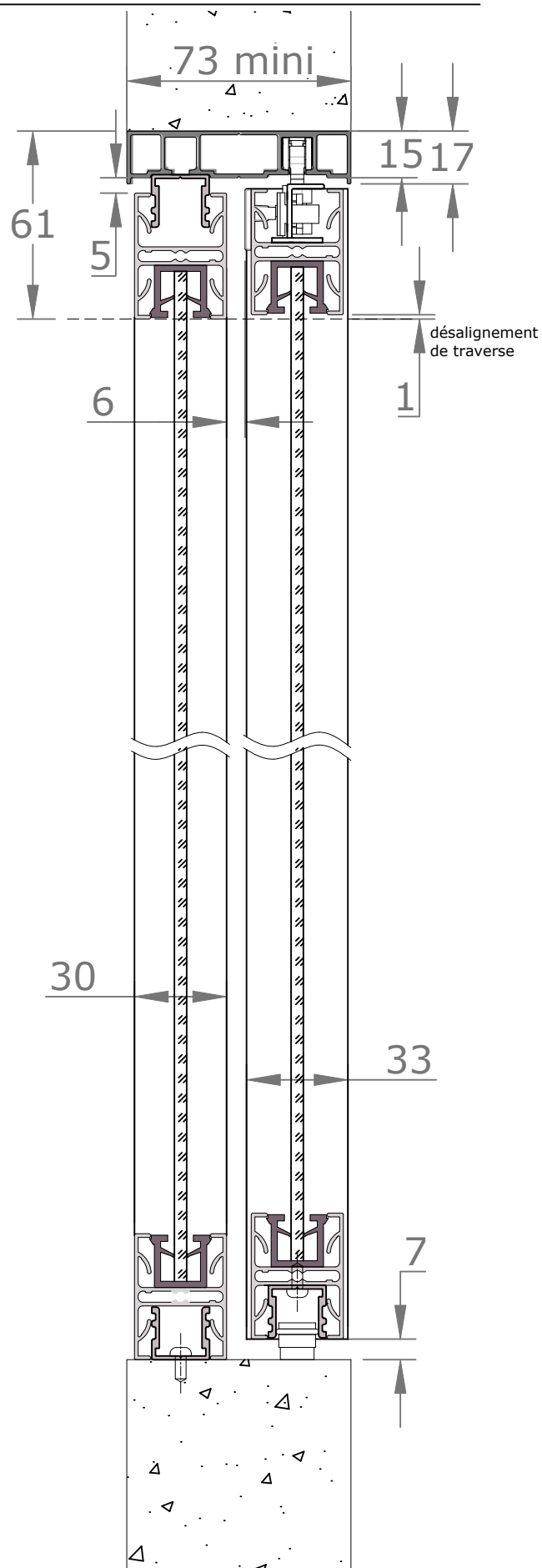
Vantail coulissant + verrière fixe
