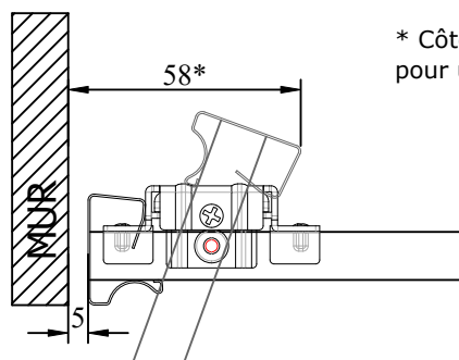
Vue: Coupe
