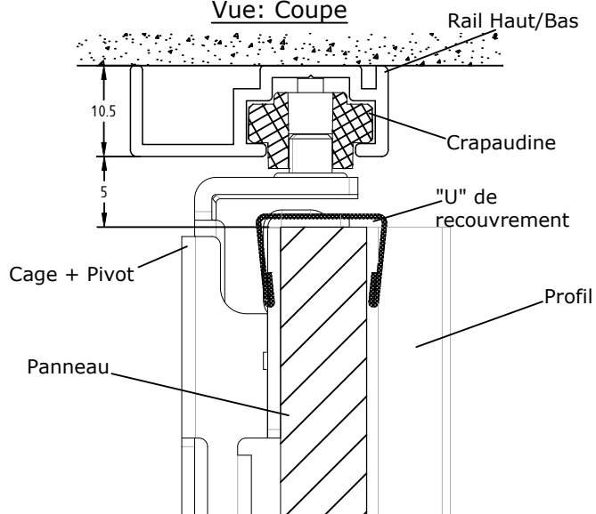
Vue: Coupe
