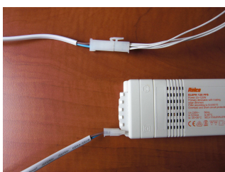
Connexion du luminaire vers le câble et du câble vers le Transfo.
