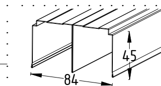
Rail Haut: -Acier laqué ou enrobé -Longueur maxi : 5450 mm
